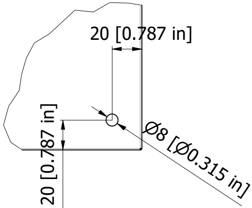
F ( 0,40 : I )
