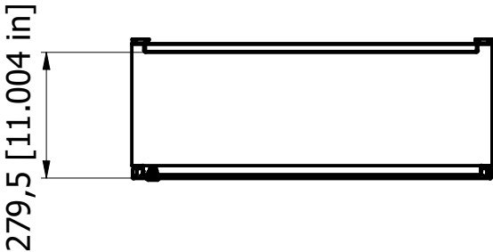
E-E ( 1 / 15 )
