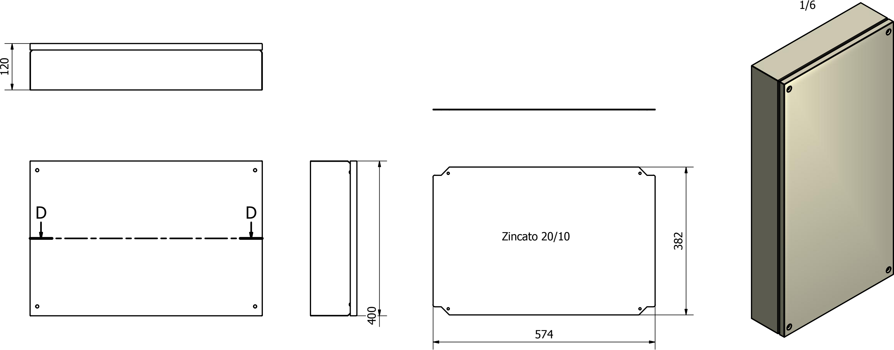
D-D ( 1 : 6 )
